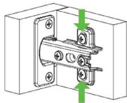
REGOLAZIONE VERTICALE
