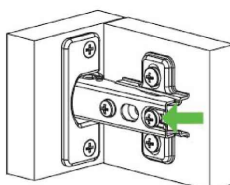
REGOLAZIONE FRONTALE
