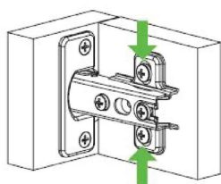
REGOLAZIONE VERTICALE
