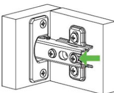
REGOLAZIONE FRONTALE
